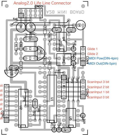
40key mod
