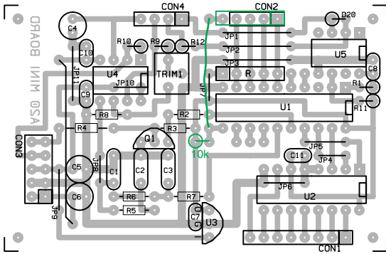
40key mod
